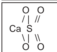
CaSO 4 Solfato di Calcio (Gessi)
