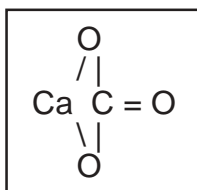
CaCO 3 Carbonato di Calcio (marmi)
