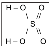
\text{H}_2\text{SO}_4 acido solforico
